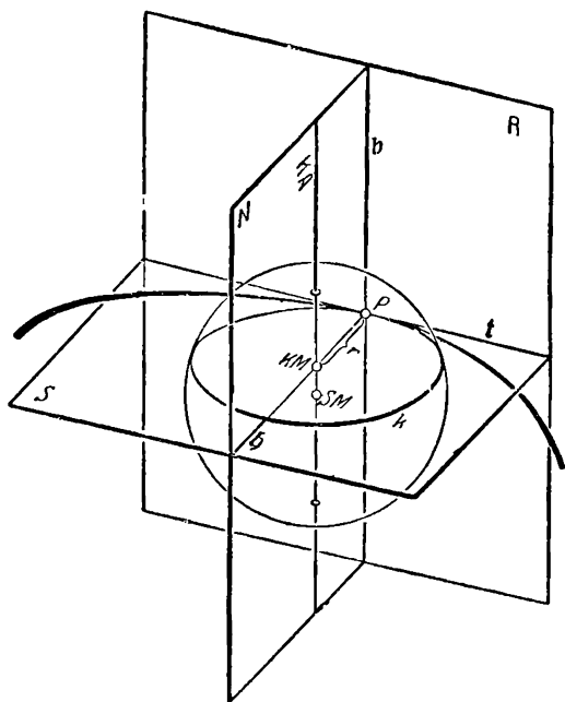
Черт. 189. P — рассматриваемая точка кривой; S — соприкасающаяся плоскость; N — нормальная плоскость; R — спрямляющая плоскость; t — касательная; h — главная нормаль; b — биномаль; k — круг кривизны; r — радиус кривизны; KA — ось кривизны; KM — центр кривизны; SM — центр соприкасающегося шара.
