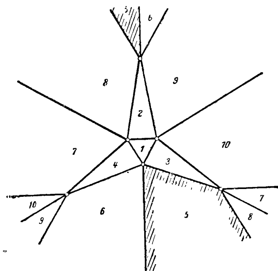
Черт. 168. Икосаэдр.
