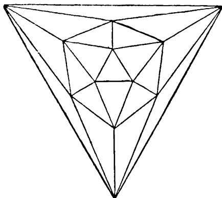
Черт. 157. Икосаэдр.
