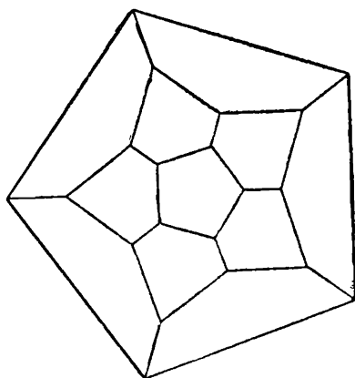
Черт. 156. Додекаэдр.
