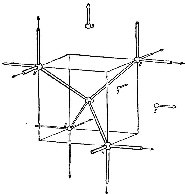
Черт. 174б. 8-ячейка.
