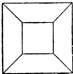
Черт. 154. Куб.
