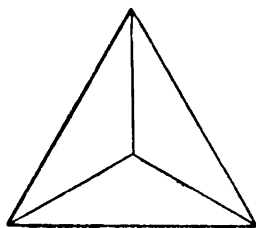
Черт. 153. Тетраэдр.
