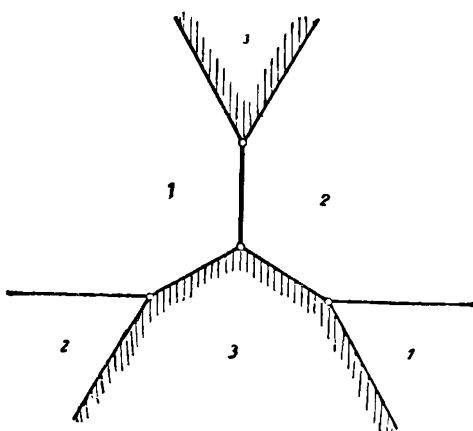
Черт. 161. Куб.
