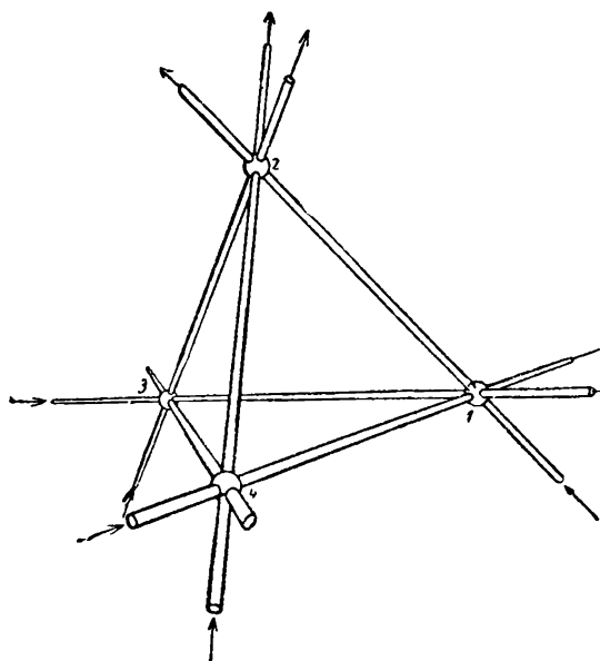
Черт. 173а. 16-ячейка.
