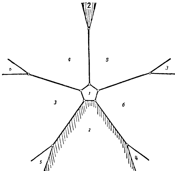
Черт. 167. Додекаэдр.
