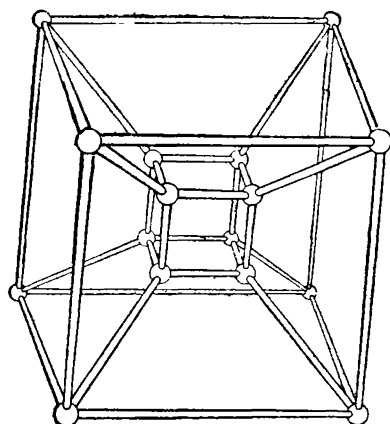
Черт. 170. 8-ячейка.
