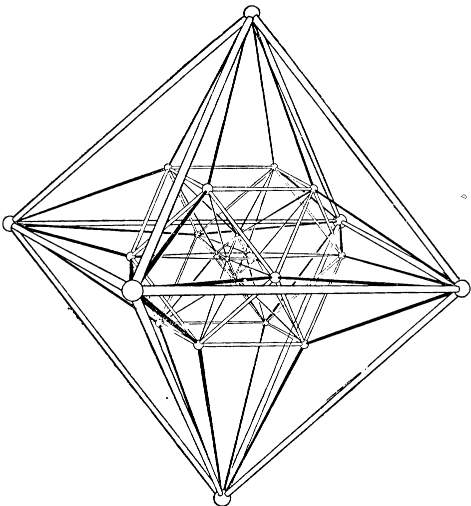
Черт. 172. 24-ячейка.
