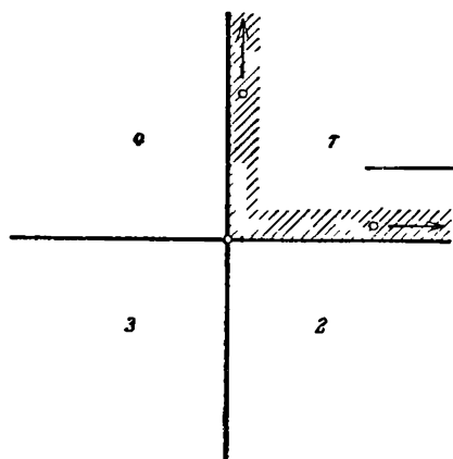
Черт. 160. Октаэдр.
