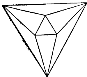
Черт. 155. Октаэдр.
