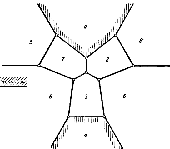
Черт. 162. Додекаэдр.
