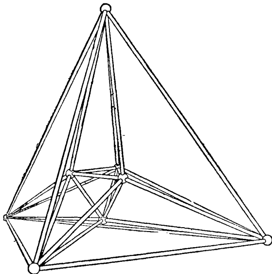
Черн. 171. 16-ячейка.
