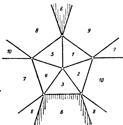
Черт. 163. Икосаэдр.
