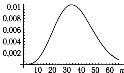
График P_{365}(n) - \tilde{P}_{365}(n)
