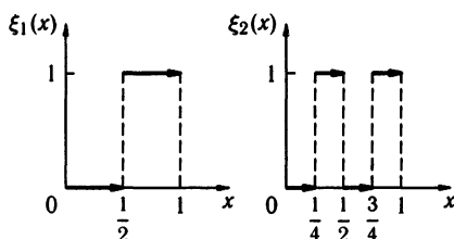
Рис. 30. Бернуллиевские величины
