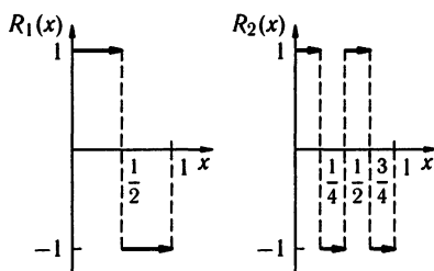
Рис. 31. Функции Радемахера
